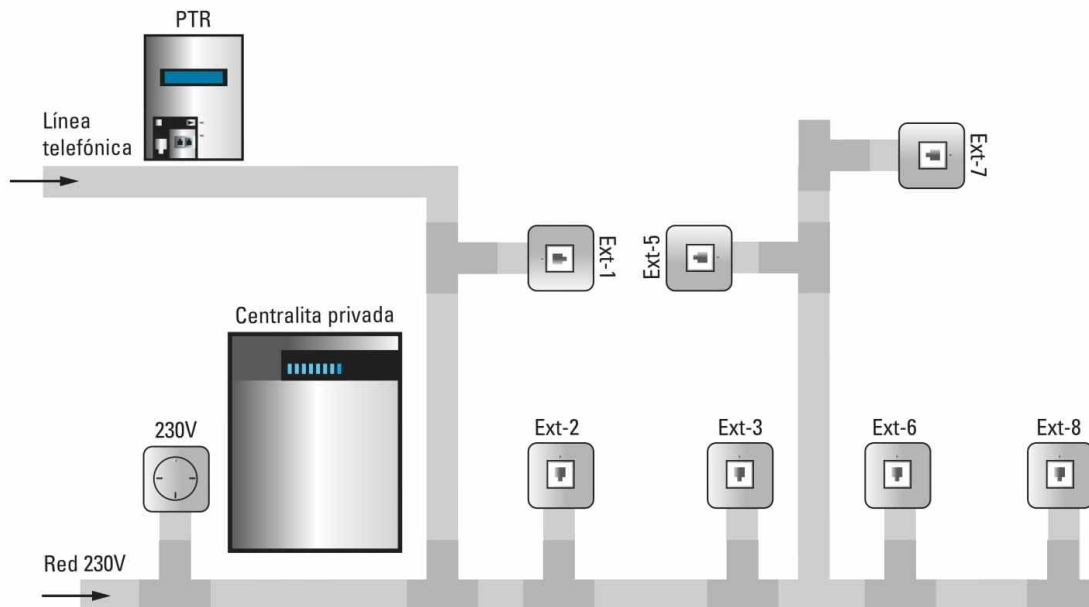
Instalación de una central telefónica analógica. Observemos la instalación interior realizada con canaletas de superficie (cable canal).
