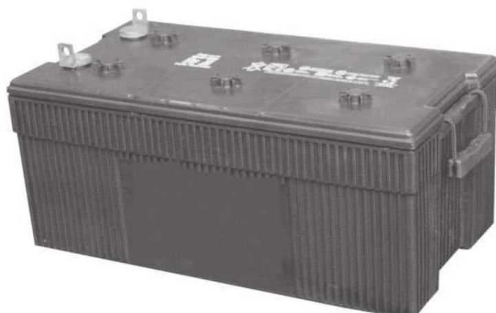
Batería de plomo-ácido de 150 Ah optimizada para sistemas fotovoltaicos con placas más gruesas, más electrolito, no son selladas y con mantenimiento bajo de 1-2 veces/año.
