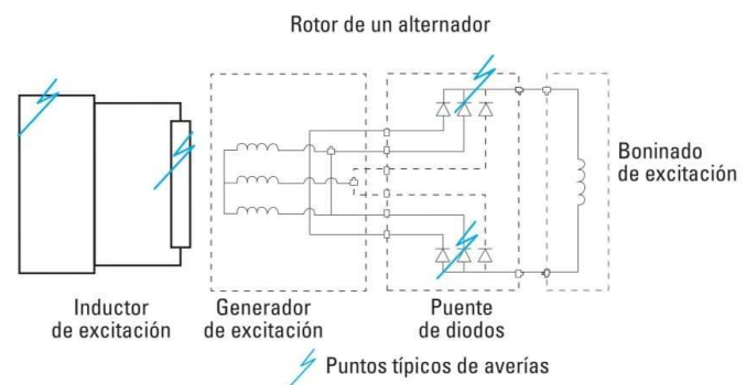
Puntos típicos de falla en el alternador de un grupo electrogénico.
