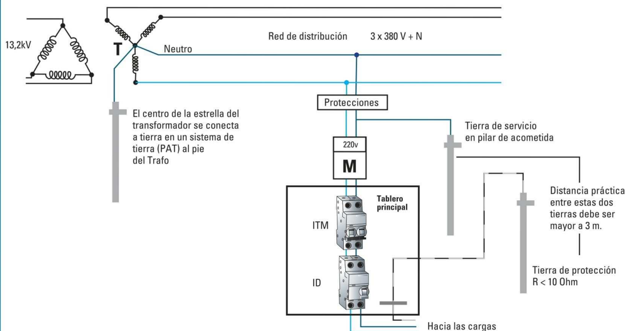
Esquema de tierra obligatorio para el suministro eléctrico. Debe ser inspeccionado para otorgar la conformidad de la instalación.
