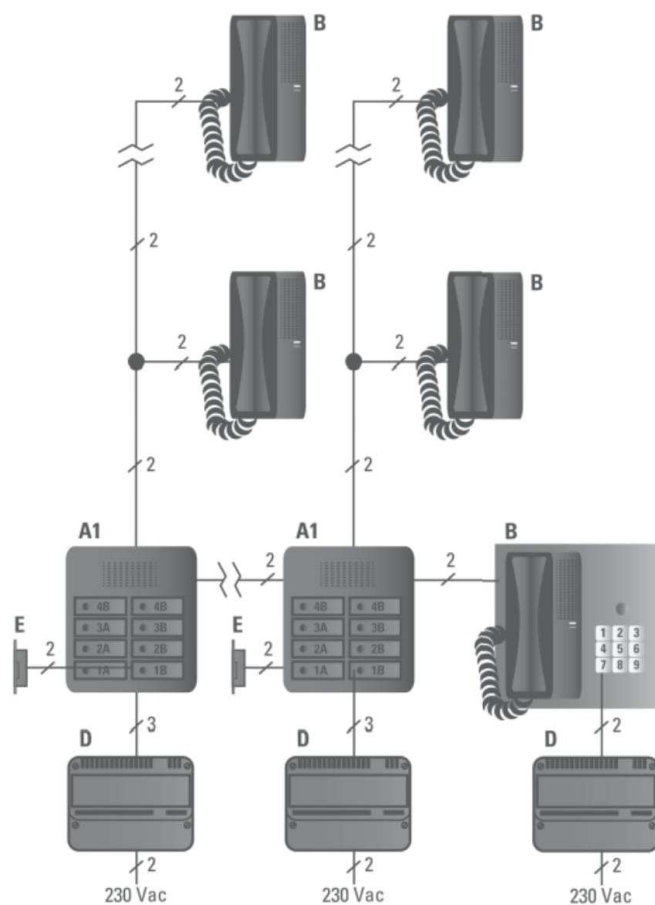
Instalación de un portero digital de dos hilos (red), que incluye una placa principal y dos o más placas secundarias con grupo fónico de red.
