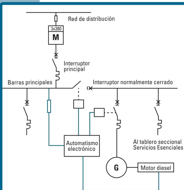
Esquema de un tablero principal para ingreso automático de GE con barras partidas, que divide servicios esenciales de no esenciales.
