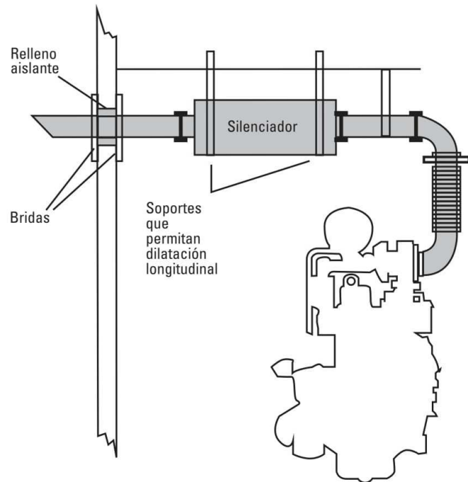
Instalación de un caño de escape de un motor primario. Puntos por verificar en inspecciones periódicas.
