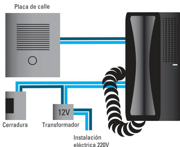
Ejemplo de un montaje 2 + 2 hilos con cableados que separan la placa de calle-telefono, de la cerradura-fuente de alimentación-telefono.
