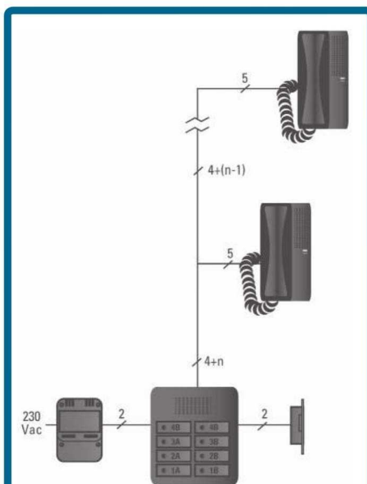
En un sistema portero convencional, la llamada en una vivienda se genera presionando el pulsador adecuado en la placa de calle.
