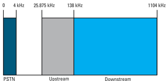
Plan de frecuencias en ADSL (Asymmetric Digital Subscriber Line), una tecnología de acceso a Internet de banda ancha mediante línea de abonado.
