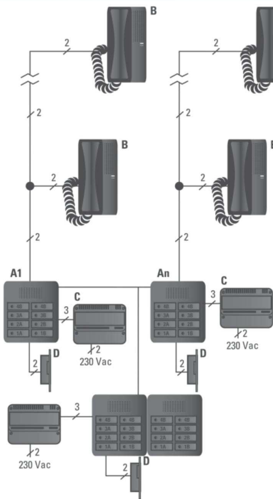
Esquema de la instalación de un portero digital de dos hilos (red) que incluye una placa principal y dos o más placas secundarias.
