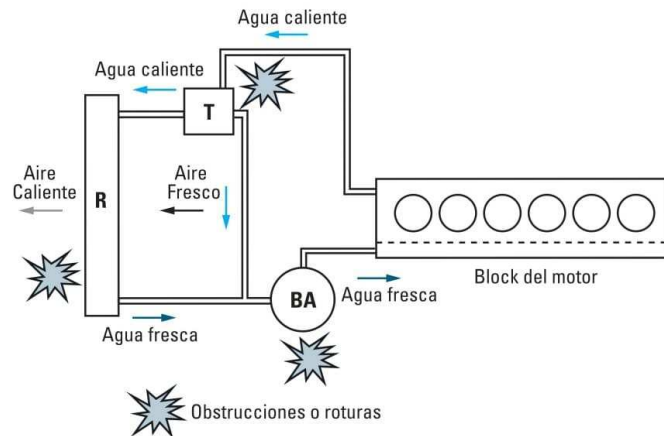
Circuito de refrigeración de una máquina motriz. Se indican los puntos típicos de falla ante calentamiento.
