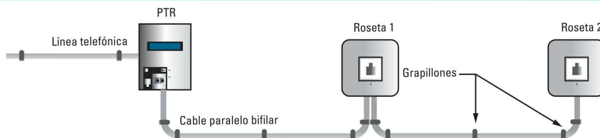
Instalación telefónica interna básica a partir de un PTR y roseta sobre pared. Es importante conservar la prolijidad al efectuar la instalación.
