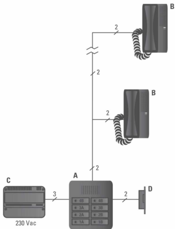
Esquema de un portero digital de dos hilos y una puerta, donde se observan los materiales requeridos para efectuar la instalación.
