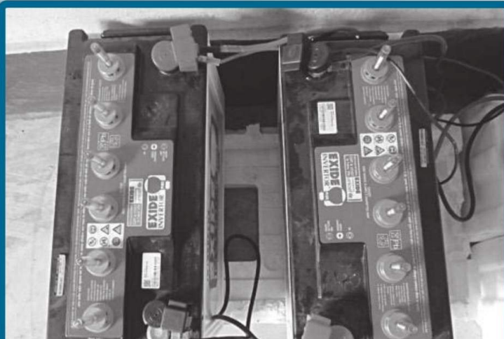
Paso 5: instalación de la batería. Instalaremos la batería sobre una base aislada en un lugar protegido de la intemperie, seco y ventilado.
