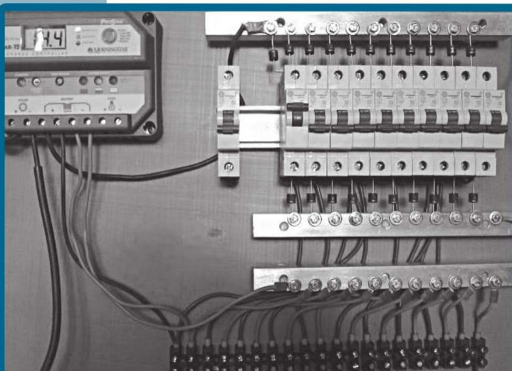
Paso 7: elementos de protección para la instalación fotovoltaica. Debemos utilizar diodos de protección para bloquear la descarga de la batería, y de bypass en los módulos fotovoltaicos.
