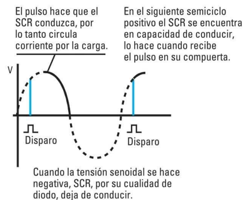
Esquema de funcionamiento de un SCR (tiristor). El semiconductor conduce cuando recibe un pulso en su compuerta.
