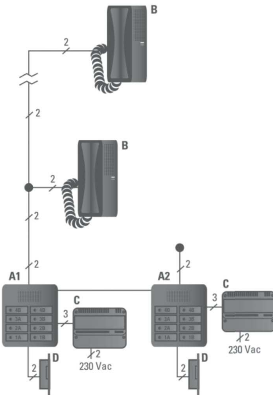
Esquema de la instalación de un portero digital de dos hilos y dos puertas de acceso (red), que incluye un grupo fónico digital con red.
