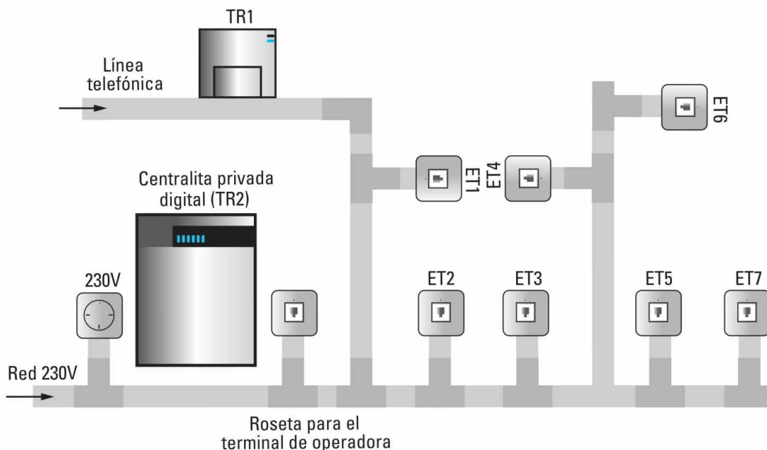
En este diagrama podemos observar la instalación de una central telefónica digital.
