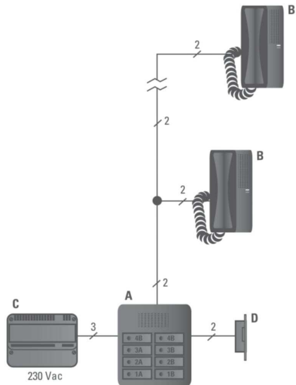
Esquema de la instalación de un portero digital de dos hilos y una puerta de acceso (red), que incluye un grupo fónico digital con red.
