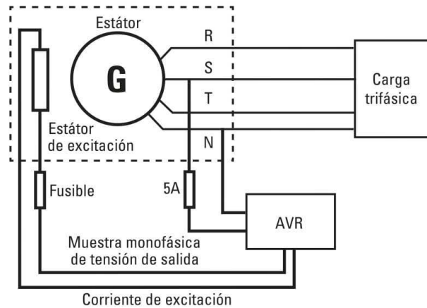
Esquema de conexión de un AVR. Se toma una muestra de tensión monofásica y se controla la excitación según varíe la tensión.
