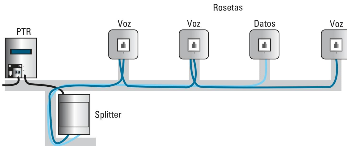
Detalle de la conexión compartida de voz y datos ADSL. Seleccionar colores diferentes facilita la instalación y su mantenimiento.
