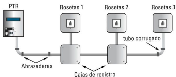
Cómo instalar una red telefónica interna desde un PTR mediante rosetas empotradas. Debemos conservar la limpieza al instalar los elementos.
