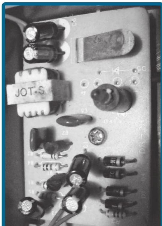
Placa que contiene la electrónica discreta para la fuente de alimentación y etapa de audio en un portero eléctrico convencional.
