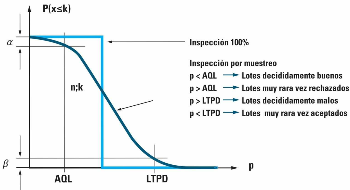
Comparación de la Curva de Inspección al 100 % con la Curva de Inspección por muestreo.
