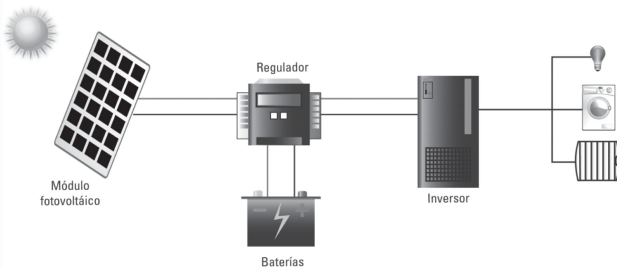
Esquema general en bloques para una instalación fotovoltaica totalmente aislada de la red de distribución eléctrica estándar.
